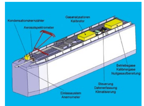
Abb. 2 Karlsruher AEROTRAM mit Instrumentierung für meteorologische und luftchemische Messungen auf dem Wagendach.
