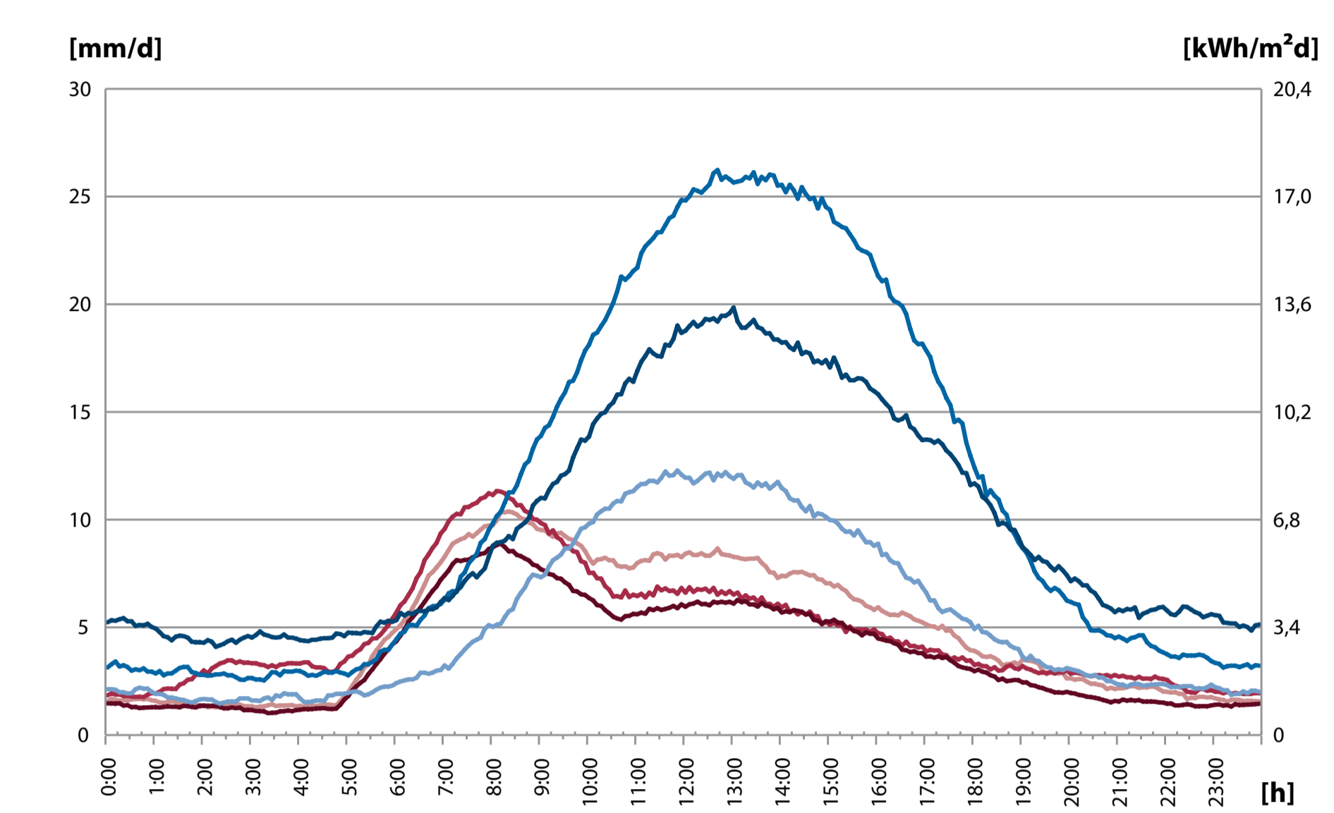
Reale Verdunstung einer Fassadenbegrünung aus Pflanzkübeln, Durchschnittlicher Tagesverlauf des Wasserbedarfs einer Anstaubbewässerung im Zeitraum von 2 Sommermonaten (mm/Tag sowie Verdunstungsäquivalent in kWh)
